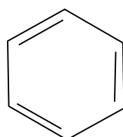
Fórmula de bastão
