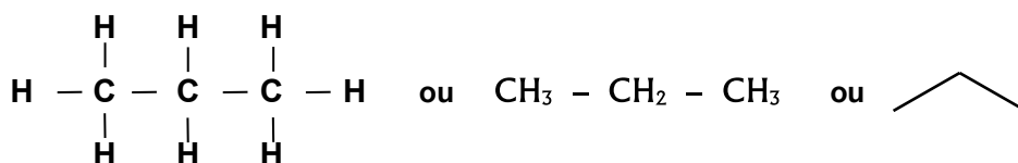
Fórmula estrutural expandida
