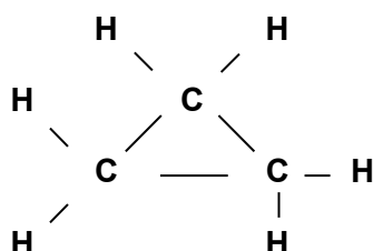
Fórmula estrutural expandida
